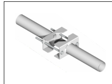
AD1702W sbraccio pesante doppio d. 60 x 250 mm orizzontale per palo d. 60 ÷ 105 mm
