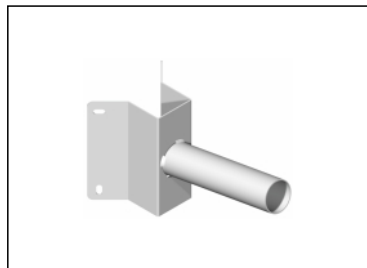
SB4110W sbraccio d. 60 x 250 mm inclinato 10° da angolo parete
