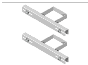
coppia supporti INOX naturale per fissaggio quadri elettrici CQ1223X l. 230 mm int. 86 ÷ 210 CQ1230X l. 300 mm int. 158 ÷ 278 CQ1240X l. 400 mm int. 218 ÷ 378 CQ1250X l. 500 mm int. 318 ÷ 478
