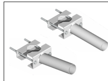
sbracci pesanti d. 60 x 250 mm per palo d. 60 ÷ 105 mm
