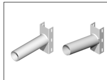
sbracci d. 60 x 220 mm per palo d. 70 ÷ 300 mm
